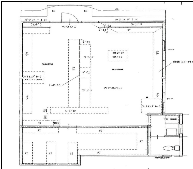
1階平面図
